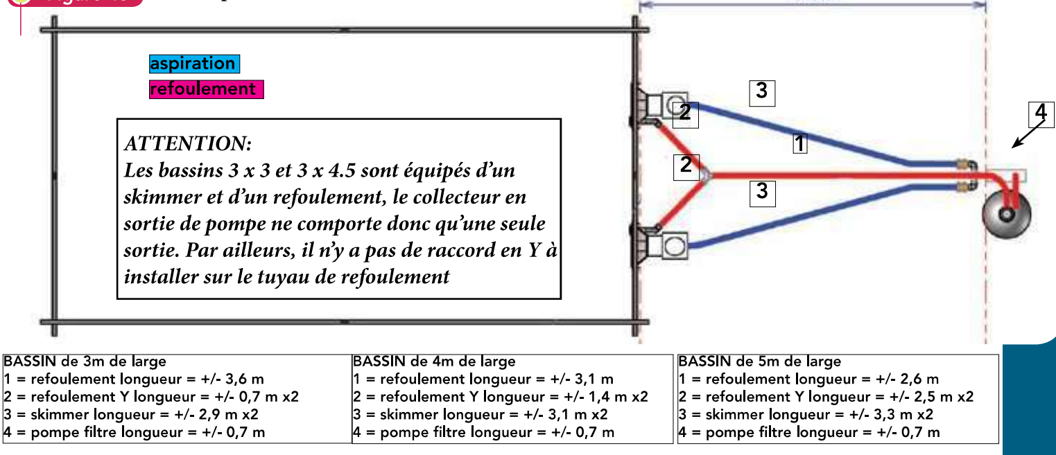
Figure 45 Exemple de filtration avec deux skimmers
