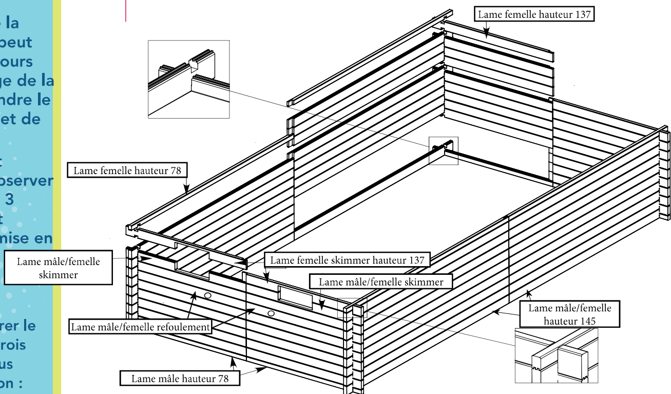
Figure 10 EMPLACEMENT DES LAMES PAR TYPE
